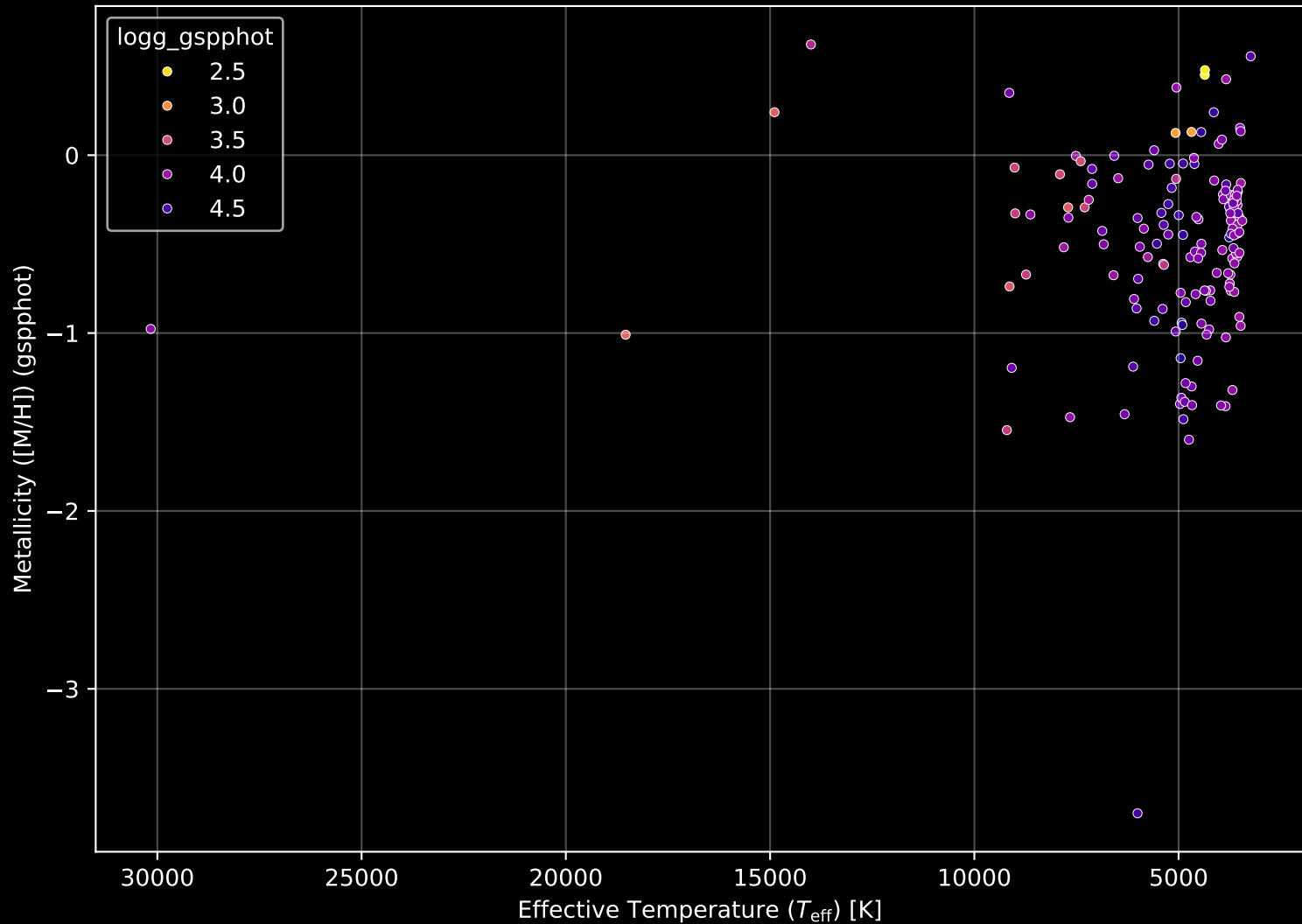
APOGEE DR17 Field: [265+01-C] Stellar Population Parameters (n= 159)
